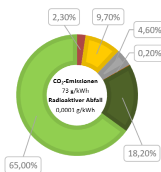
verbleibender Energieträgermix der SWG 2
