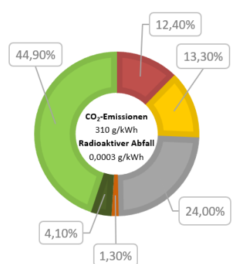
Energieträgermix für Deutschland 3
