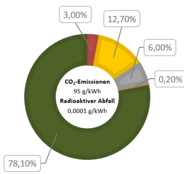
Gesamtenergieträgermix der SWG 1
